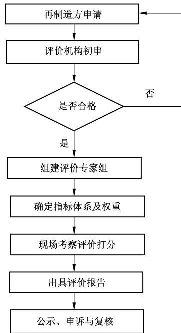
图 1 再制造机械产品质量评价流程
